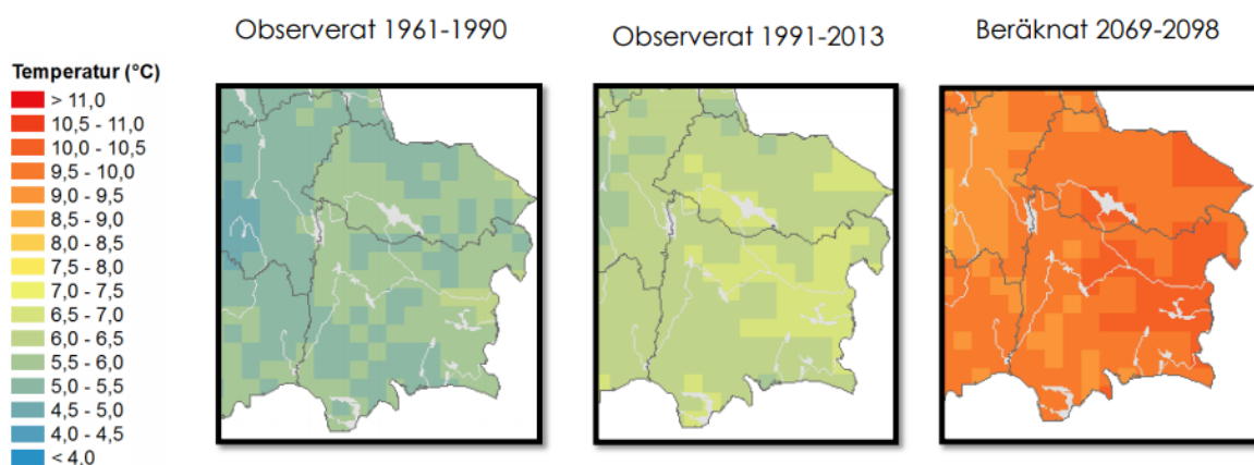
Figur 14. Källa: Länsstyrelsen i Jönköpings län 2017. Observerad och beräknad medeltemperatur i Vetlanda kommun.
