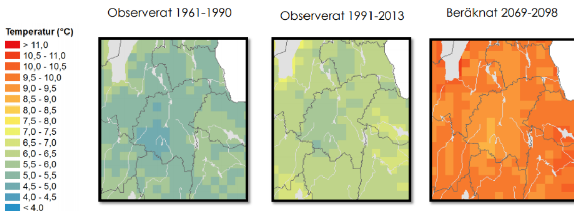
Figur 13. Källa: Länsstyrelsen i Jönköpings län 2017. Observerad och beräknad medeltemperatur i Nässjö kommun. Under åren 1961 till 1990 var medeltemperaturen i Nässjö kommun 4 till 5 grader. Mellan 1991 till 2013 steg medeltemperaturen till 5 till 6 grader. Enligt Länsstyrelsens beräkningar så kommer medeltemperaturen vara mellan 8 och 9 grader mellan åren 2069–2098.
